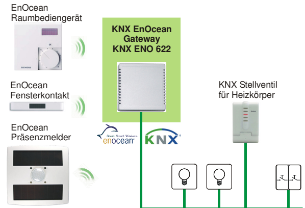
Abbildung 5: Anwendungsbeispiel Heizungsregler
