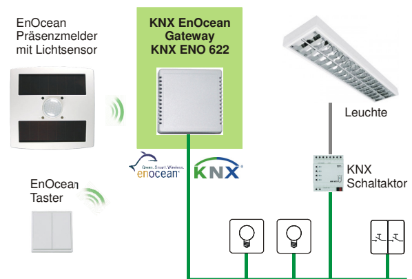
Abbildung 6: Anwendungsbeispiel Lichtsteuerung
